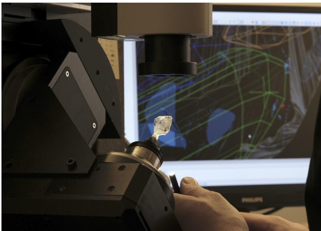
Toestel om de insluitsels in diamant in kaart te brengen, Diamcad , 2025
